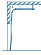
Höhergeführter Laufschienenbeschlag
