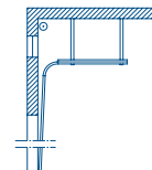
wie Beschlagsart H mit höherliegender Torsionsfederwelle
