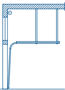
wie Beschlagsart N mit höherliegender Torsionsfederwelle
