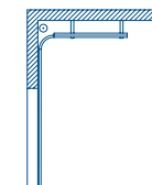
wie Beschlagsart H mit steiler Laufschiene und Schlitzbreite mind. 120 mm (für Verladerrampen-Tore) Torbreite LZ ≤ 3500 mm Torhöhe RM ≤ 5000 mm Nicht möglich bei den Tortypen ASP40/ASR40/ALS40 und Toren mit Schlüpfür sowie mit Echtglasfüllung!
