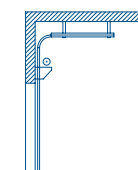
wie Beschlagsart HU mit steiler Laufschiene und Schlitzbreite mind. 120 mm (für Verladerrampen-Tore) Torbreite LZ ≤ 3500 mm Torhöhe RM ≤ 5000 mm Nicht möglich bei den Tortypen ASP40/ASR40/ALS40 und Toren mit Schlüpfür sowie mit Echtglasfüllung!
