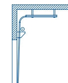
wie Beschlagsart NH mit Dachfolge (maximal 27°)
