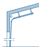
wie Beschlagsart H mit Dachfolge
